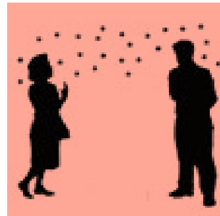
aerosols
